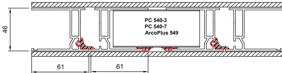
Schnitt B - B
